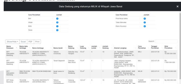
GAMBAR 28
