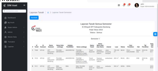
GAMBAR 25
