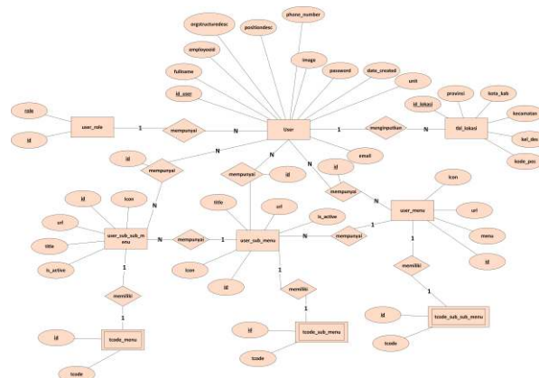
GAMBAR 4 ERD
