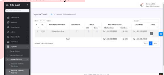
GAMBAR 27
