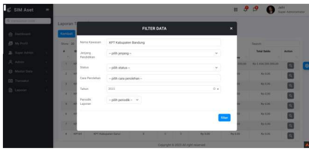
GAMBAR 22
