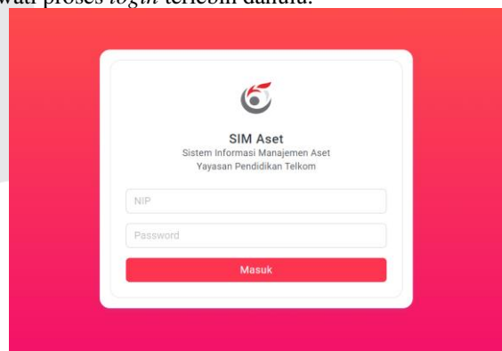
GAMBAR 6 Implementasi Login
