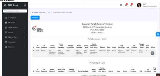
GAMBAR 24
