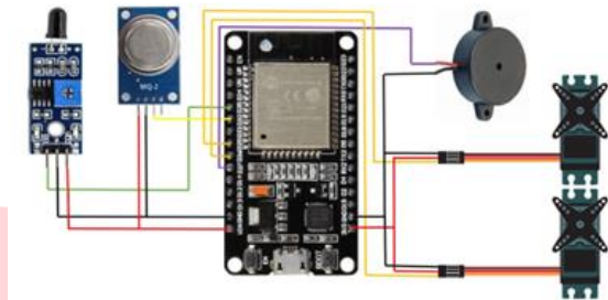
Gambar 3. 2 Perancangan Skematik
