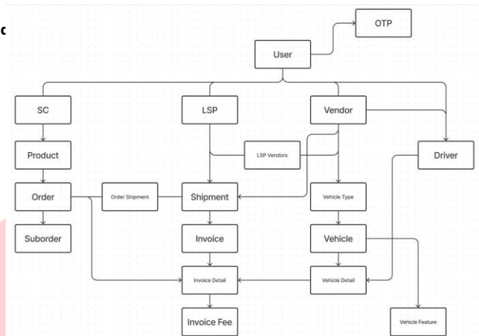
Gambar 4. 1 struktur database
