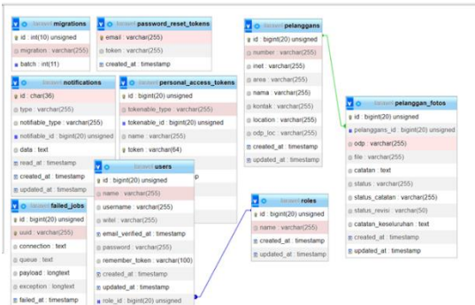
GAMBAR 3. 3 Relasi Database
