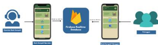
GAMBAR.1 Arsitektur Aplikasi
