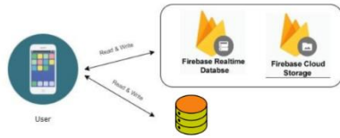
GAMBAR 3.1 Arsitektur aplikasi
