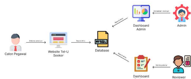
Gambar 1. Arsitektur website
