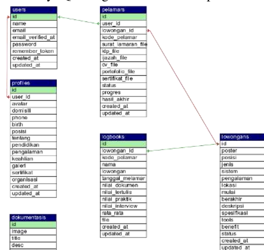
Gambar 2. Struktur Data MySQL
