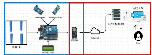
Gambar 2. 1 Gambaran sistem
