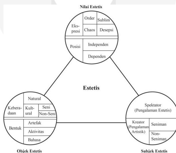
Gambar 3.1 konsep estetika
