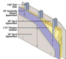
Gambar 4.6.1 Konsep Akustik
