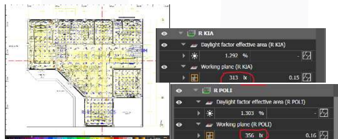
Gambar 5 Aplikasi Dialux Lantai 1
