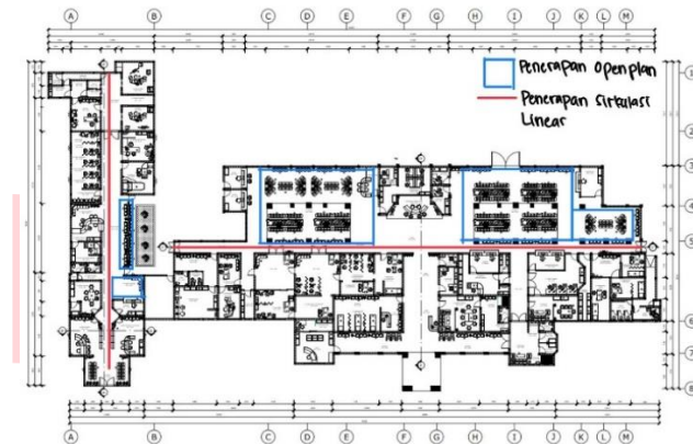
Gambar 7 Konsep organisasi ruang dan layout furniture Sumber: Dokumentasi Pribadi, 2023
