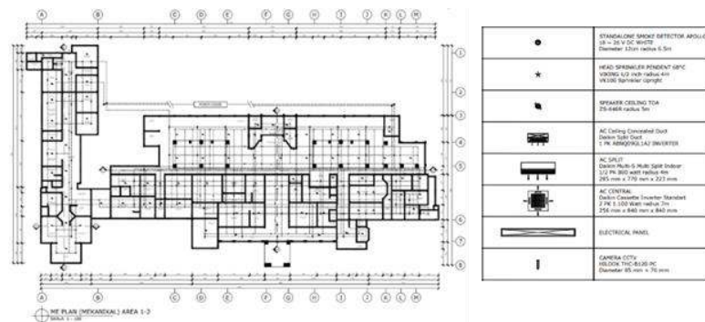
Gambar 15 Denah ME setelah perancangan Sumber: Dokumentasi Pribadi, 2023
