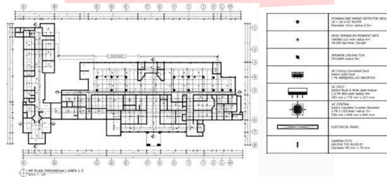
Gambar 18 Denah ME setelah perancangan Sumber: Dokumentasi Pribadi, 2023
