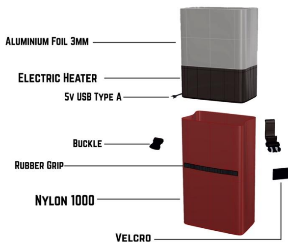
Gambar 2 Exploded View Produk Sumber: Dokumentasi Penulis
