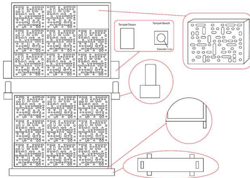
Gambar 4 Sketsa Produk (Sumber: dokumentasi penulis, 2025)
