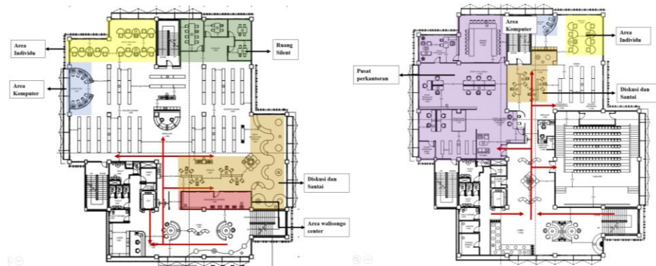
Gambar 1 Konsep Organisasi Ruang dan Layout Furnitur
