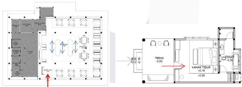
Gambar 3 Konsep Sirkulasi Sumber : Data Pribadi, 2023
