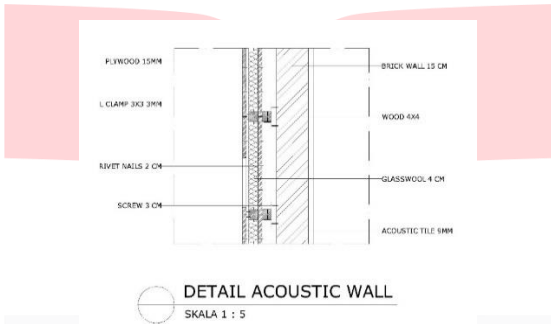
Gambar 1.14 Dinding akustik Sumber: Analisis Pribadi, 2024
