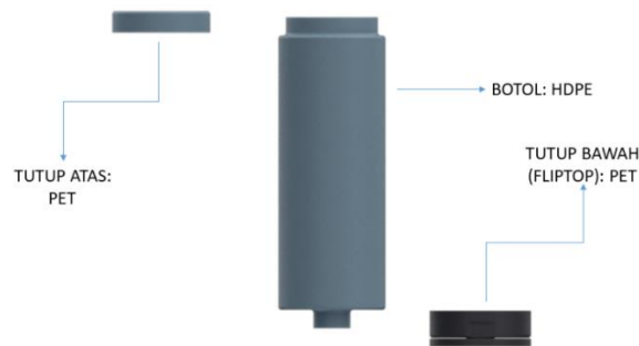
Gambar 5 Exploded View dan Skema Material Packaging Face Wash Sumber: dokumentasi penulis
