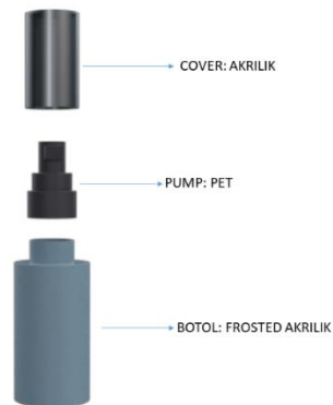
Gambar 9 Exploded View dan Skema Material Botol Serum Sumber: dokumentasi penulis
