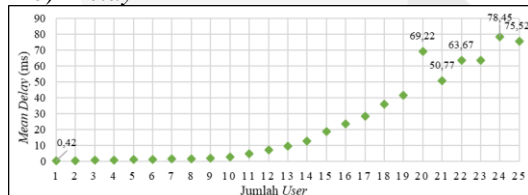
Gambar 4(a). Grafik hasil pengukuran delay skenario 1 pada API1.
