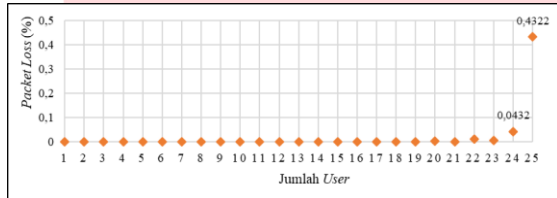
Gambar 5(a). Grafik hasil pengukuran packet loss skenario 1 pada API.
