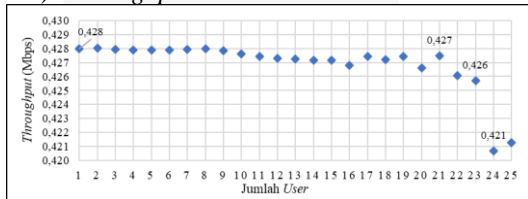
Gambar 3(a). Grafik hasil pengukuran throughput skenario 1 pada API1.
