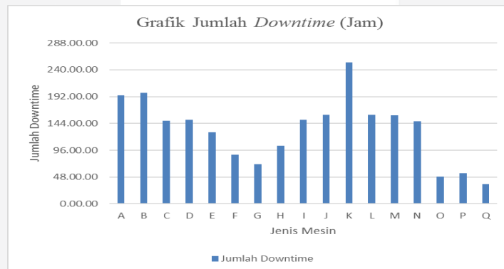
Gambar 2 Data Downtime Mesin Jet Dyeing di Unit Dyeing 6 Tahun terakhir
