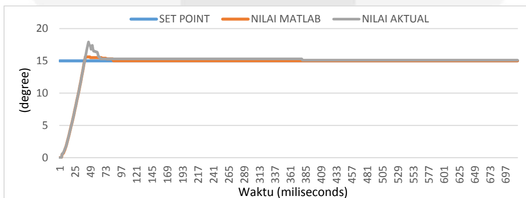
Gambar 3.5 Grafik Perbandingan Respon Sistem Aktual dan Matlab Sumbu Roll
