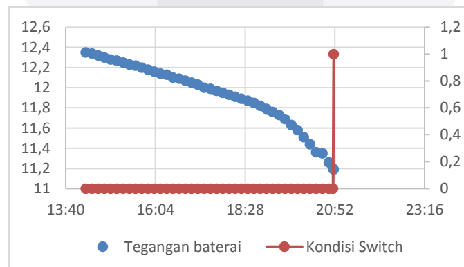
Gambar III- 1 Grafik pengujian switching saat discharging
