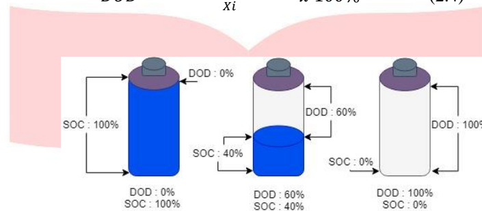
Gambar II-4. Proses DOD dan SOC
