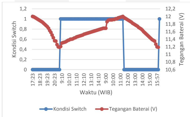
Gambar III-3. Pengujian Switching 1 siklus
