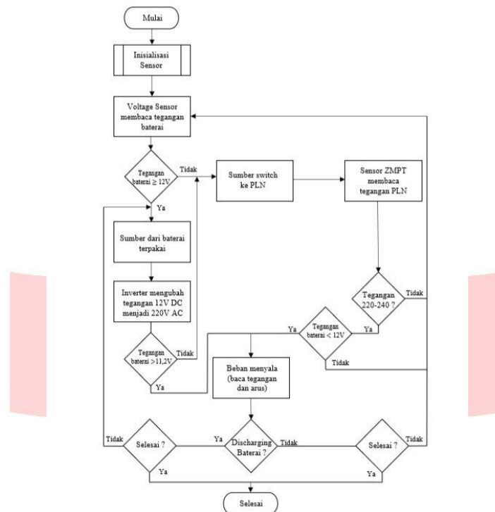
Gambar III-1. Diagram Alir Sistem
