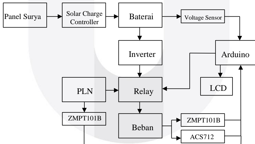
Gambar III-1. Blok Diagram Sistem Kerja Alat
