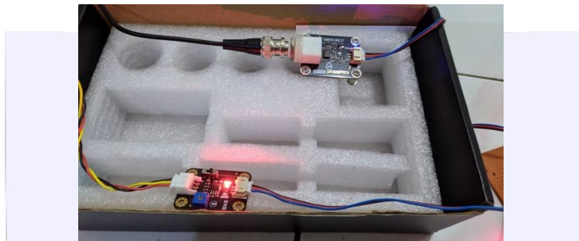
Gambar 3.1.2 Rangkaian modul sensor pH dan sensor turbidity
