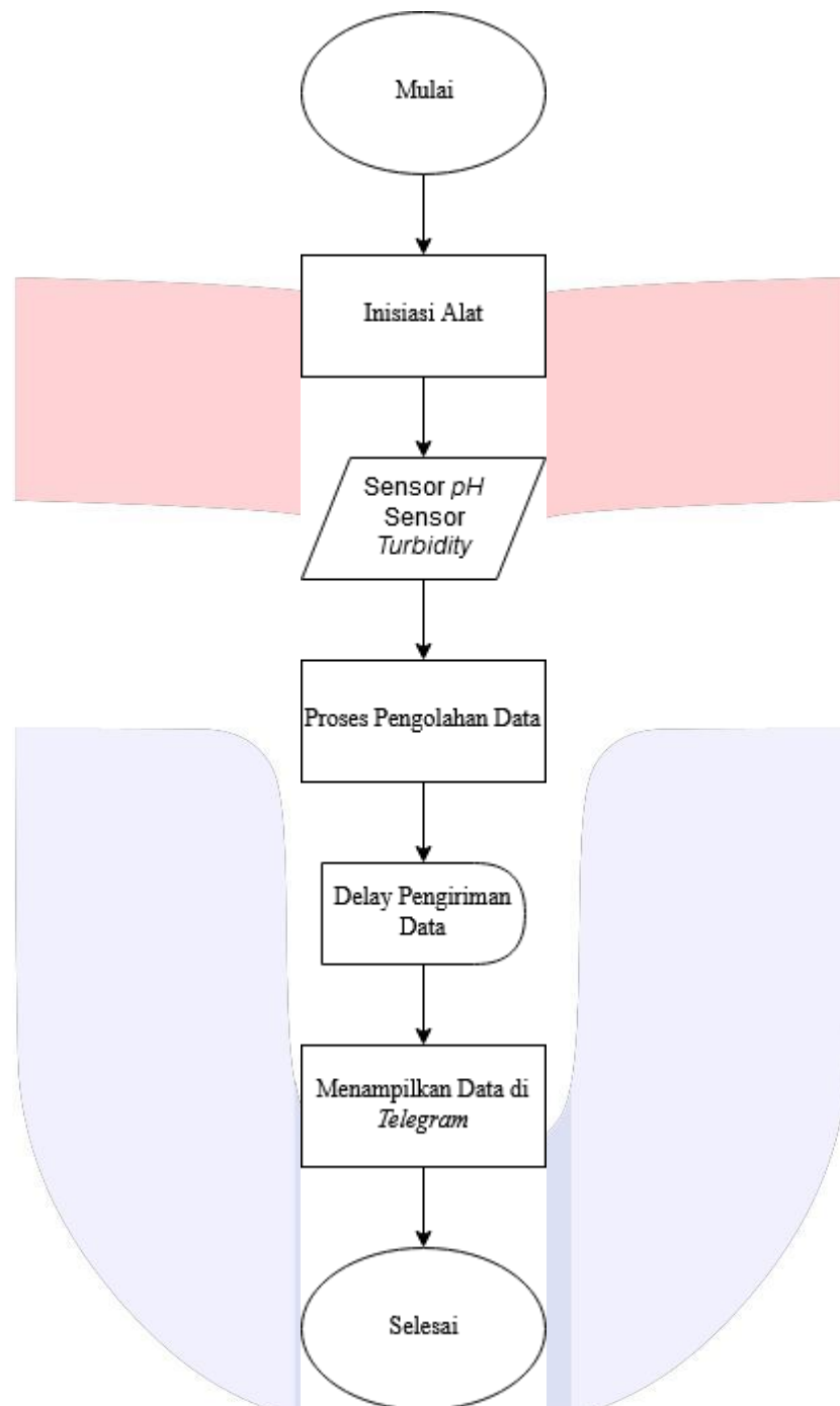
Gambar 3.2 Flowchart Alur Kerja
