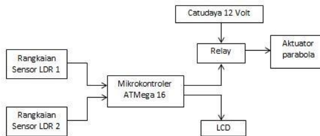
Gambar 2.3 Diagram Blok Sistem Pelacakan
