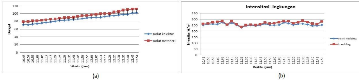
Gambar 3.4 (a) Grafik Perubahan Sudut Kolektor dan Matahari Terhadap Waktu (b) Grafik Intensitas Lingkungan
