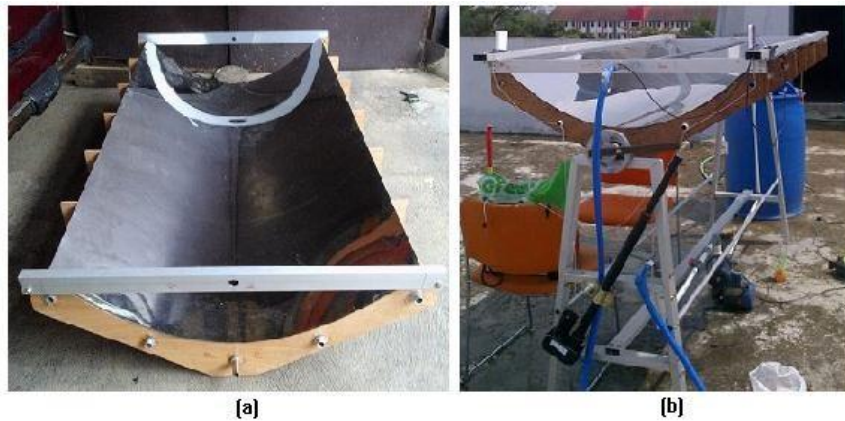
Gambar 2.2 (a) Desain Kolektor Panas (b) Kolektor Panas Dengan Aktuator Parabola
