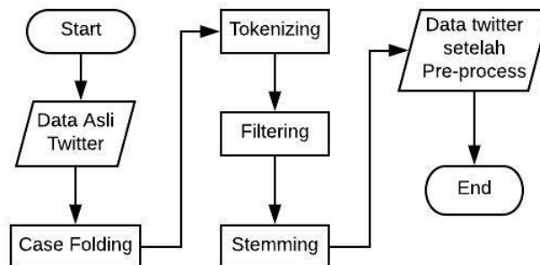
Gambar 2. Alur Proses Pada Tahap Pre-processing
