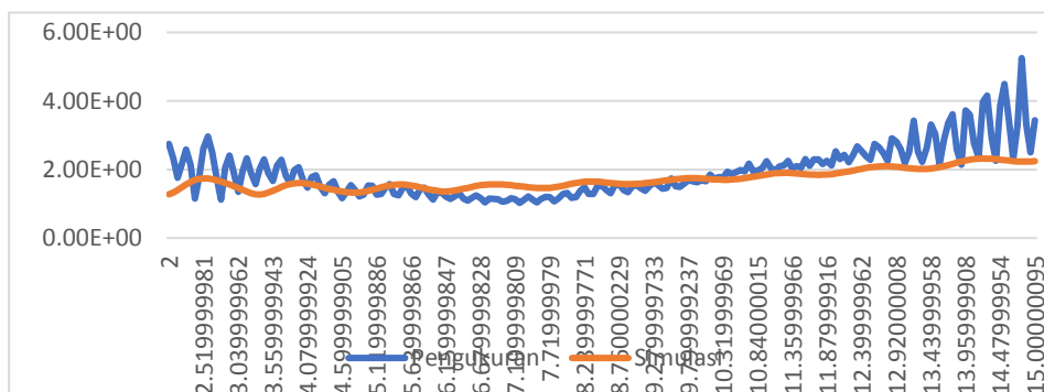
Gambar 10. Perbandingan VSWR Hasil Simulasi dan Pengukuran
