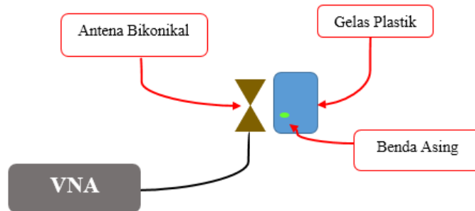
Gambar 8. Skema Pengukuran Benda Asing dengan Metode UWB.
