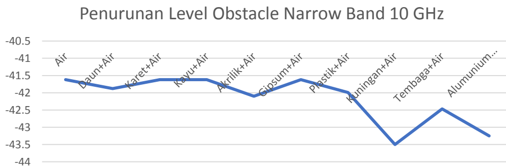
Gambar 14. Hasil Pengukuran Benda Asing 10 GHz.
