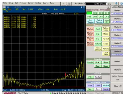
Gambar 11. Bandwidth hasil Pengukuran.
