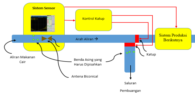
Gambar 1. Perancangan Sistem Food Radar .
