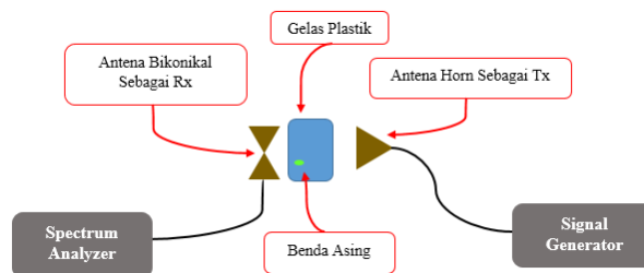
Gambar 9. Skema Pengukuran Benda Asing dengan Metode Narrow Band .
