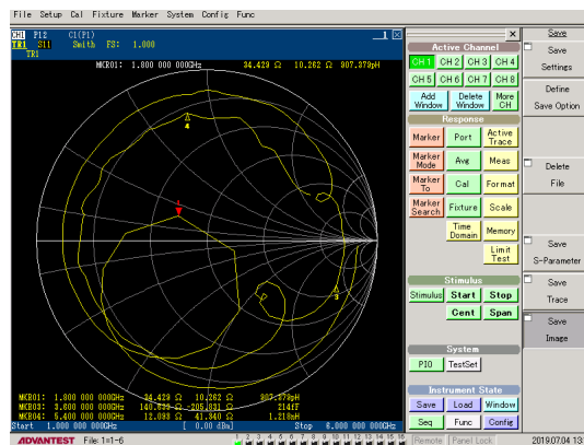
Gambar 9. Matching impedance antenna realisasi.
