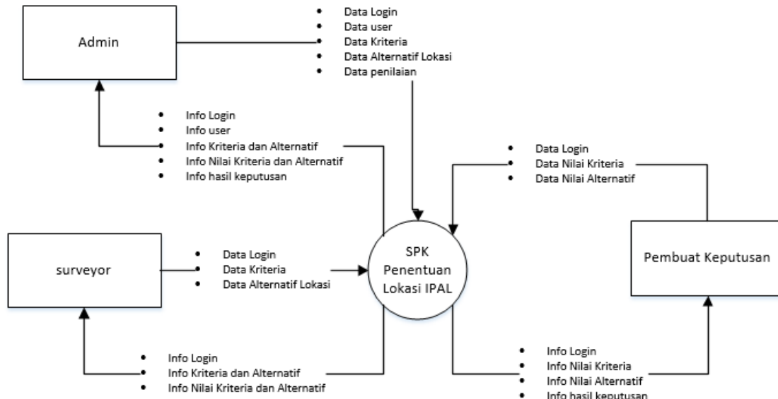
Gambar 3. Diagram Konteks
