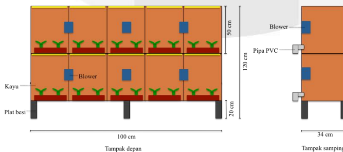
Gambar 2.5 Rancangan Alat
