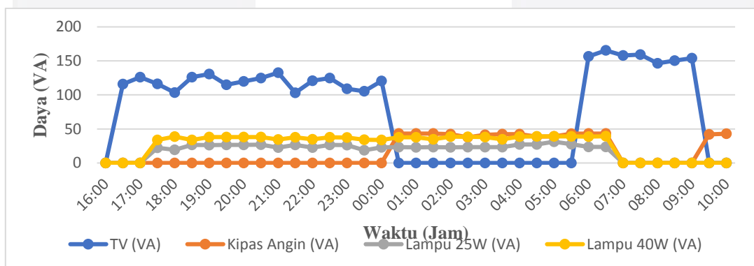
Gambar 4.2 Grafik Monitoring Arus dan Daya (VA) Peralatan Listrik
