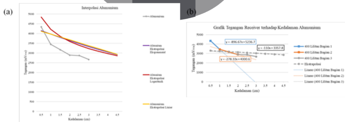
Gambar 9 Hasil ekstrapolasi pada Aluminium (a) Interpolasi Logaritmik, Ekspensial, dan Linier (b) Interpolasi Partisi Linier
