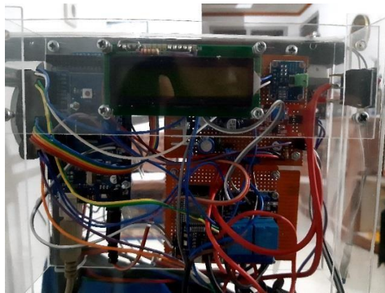
Gambar 4. 1 Implementasi Skematik Rangkaian Jemuran Otomatis
