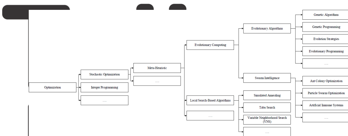
Gambar 1 Teknik Optimasi
