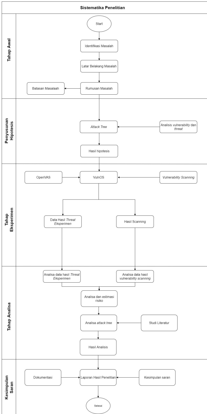
Gambar 1 Sistematika Penelitian
