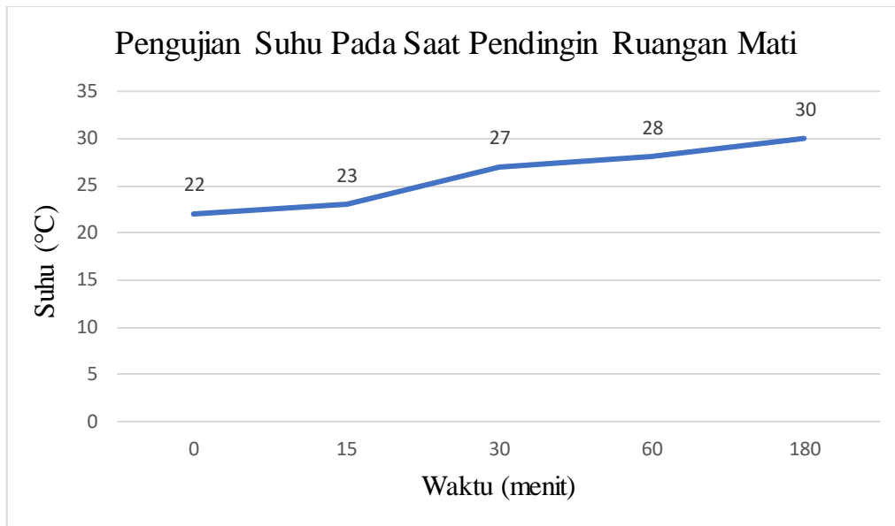
Gambar 5 Grafik Pengujian Suhu Pada Saat Pendingin Ruangan Mati
