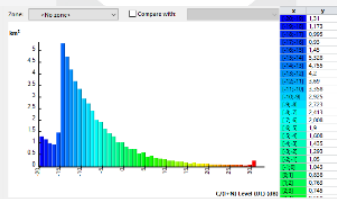
Gambar 4.51 Data hasil prediksi SNR
