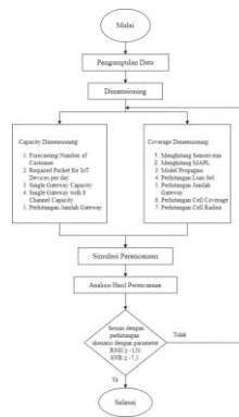
Gambar 3.1 Flowchart perencanaan LoRa
