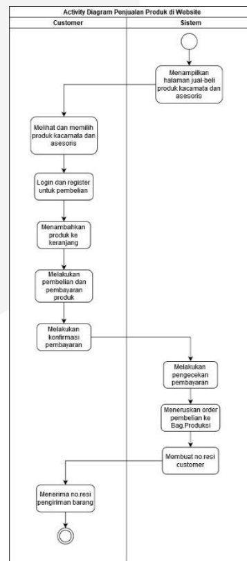
Gambar 5 Activity Diagram Penjualan Produk
