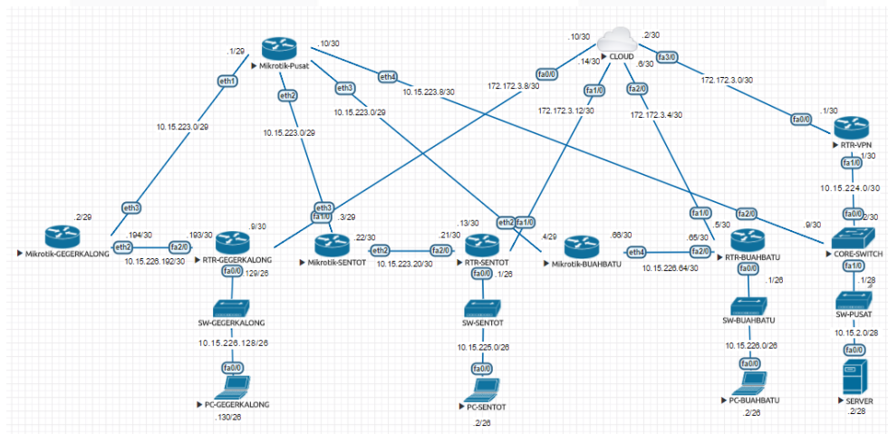
Gambar 7 Topologi simulasi jaingan nirkabel usulan metode bridging
