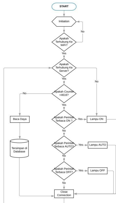
Gambar 1. Diagram Alir Sistem
