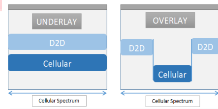
Gambar 2. 1 Representasi underlay dan overlay pada D2D [3].
