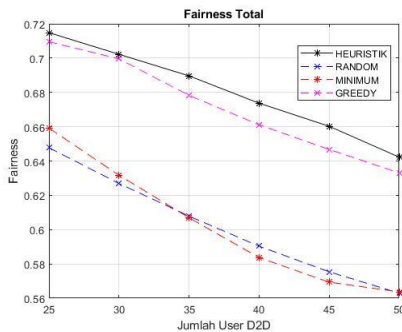
Gambar 4.7 Fairness pada skenario pertama.
