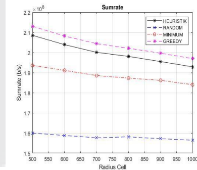
Gambar 4. 2 Sumrate total pada skenario kedua.
