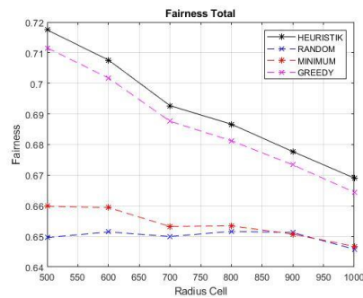
Gambar 4.8 Fairness pada skenario kedua.
