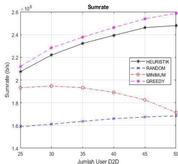
Gambar 4. 1 Sumrate total pada skenario pertama.
