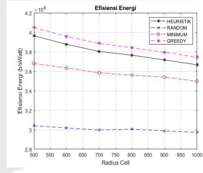
Gambar 4.6 Efisiensi Energi pada skenario kedua.
