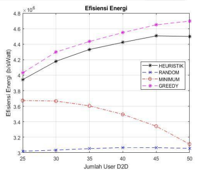
Gambar 4.5 Efisiensi Energi pada skenario pertama.
