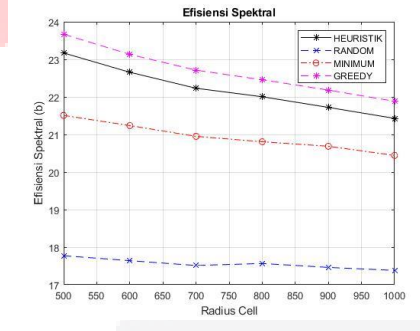
Gambar 4.4 Efisiensi Spektral pada skenario kedua.
