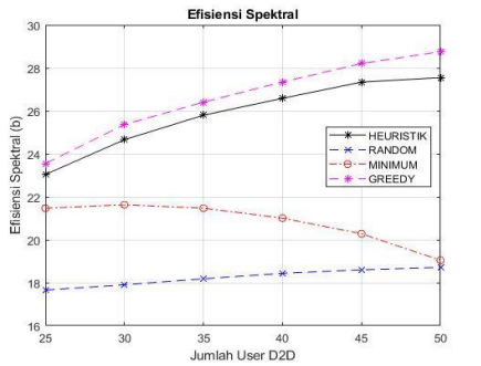
Gambar 4.3 Efisiensi Spektral pada skenario pertama.
