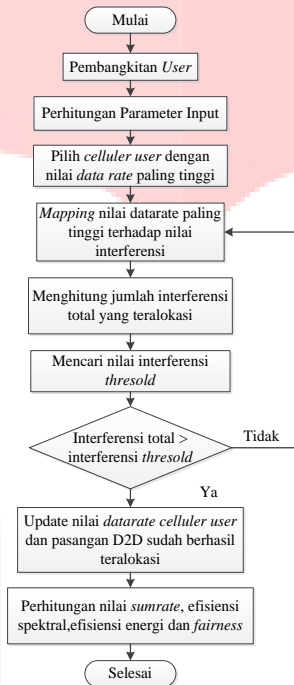
Gambar 3.3 Flowchart menjalankan Algoritma Heuristic [4]
