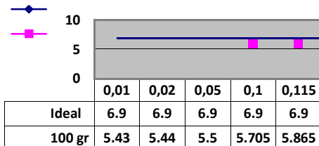
Grafik Beban 100 gr
