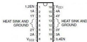
Gambar 2.6 Konstruksi Pin Driver Motor DC IC L293D
