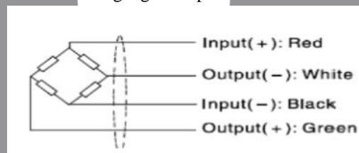
Gambar II - 1 Konfigurasi Kabel Sensor Load Cell
