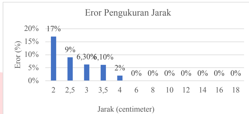
Gambar 3.1 Grafik Eror Pengukuran Jarak
