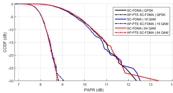
Gambar 3.8 Hasil PAPR pengujian AP-PTS terhadap pengaruh modulasi digital
