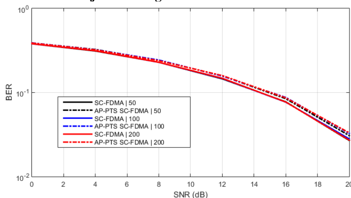
Gambar 3.15 Hasil uji BER dengan parameter jumlah partisi AP-PTS
