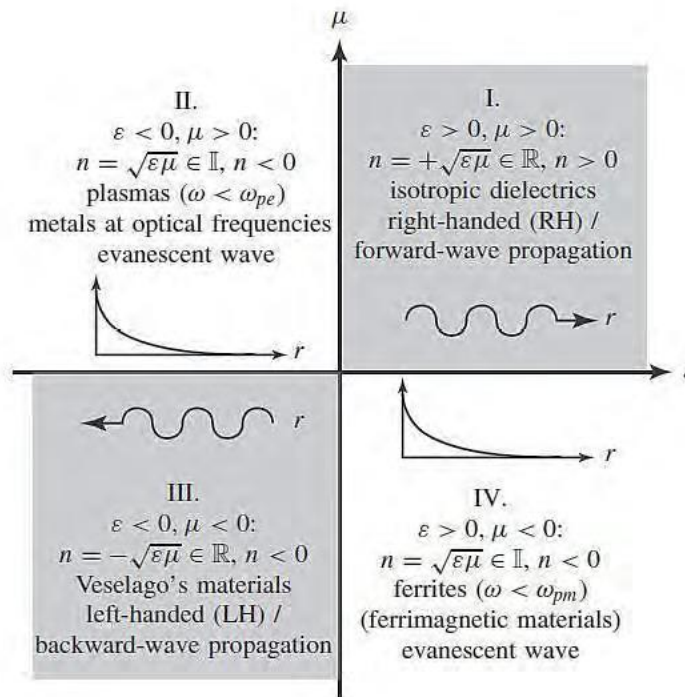
Gambar 1 Klasifikasi material[3]
