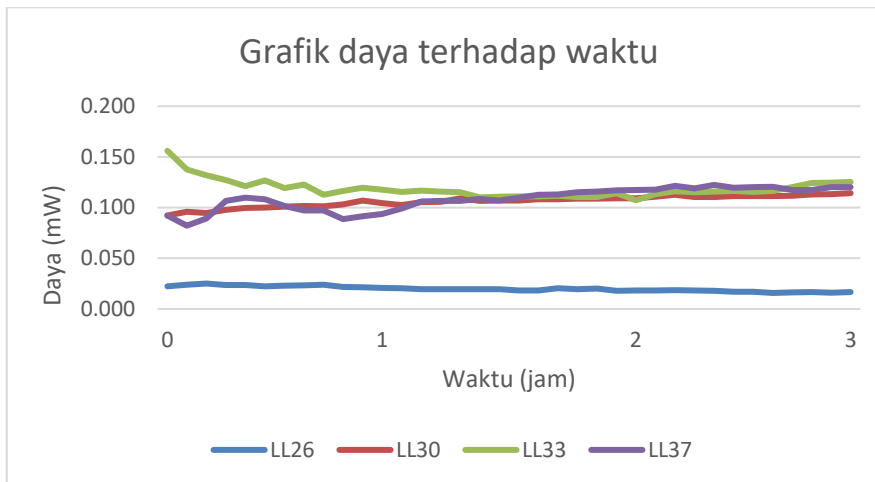
Gambar 3. Pengukuran Daya terhadap Waktu
