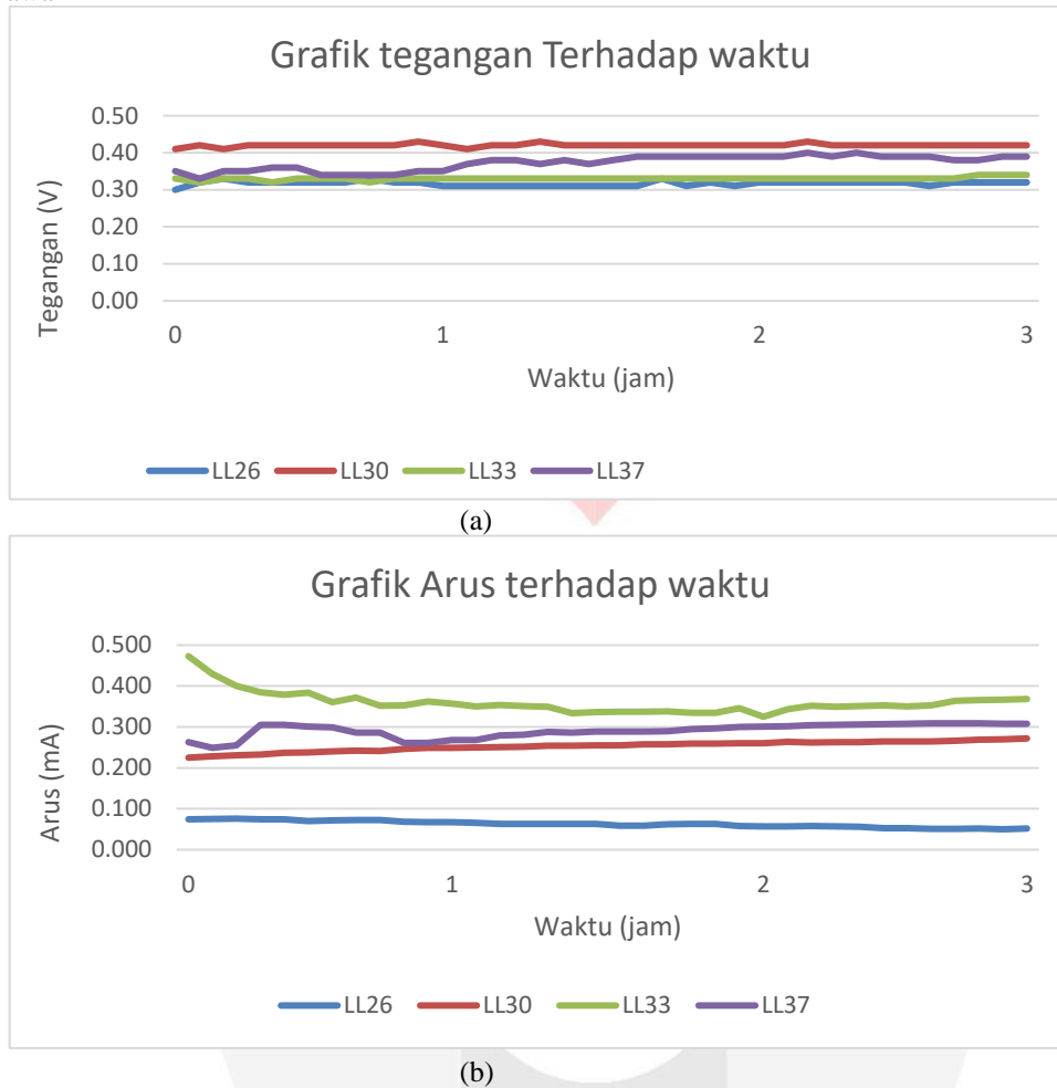
Gambar 1. (a) Pengukuran Tegangan terhadap Waktu, (b) Pengukuran Arus terhadap Waktu
