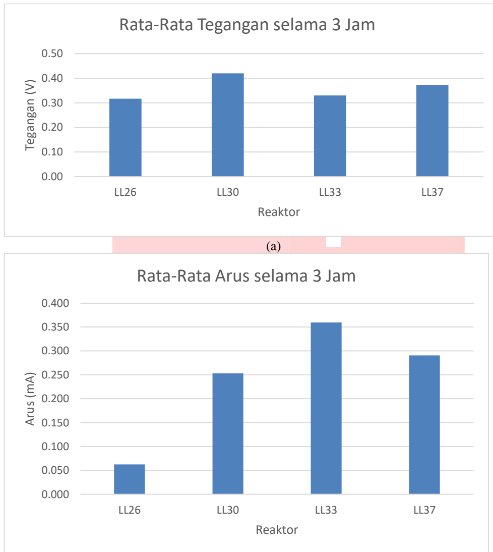
(b) Gambar 2. (a) Bagan Rata-Rata Tegangan selama 3 Jam, (b) Bagan Rata-Rata Arus selama 3 Jam
