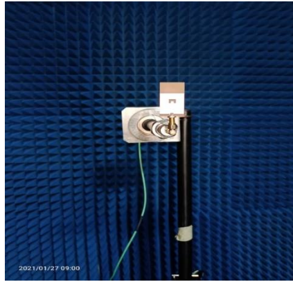
Gambar 7. Pengukuran Antena Yang Sudah Difabrikasi
