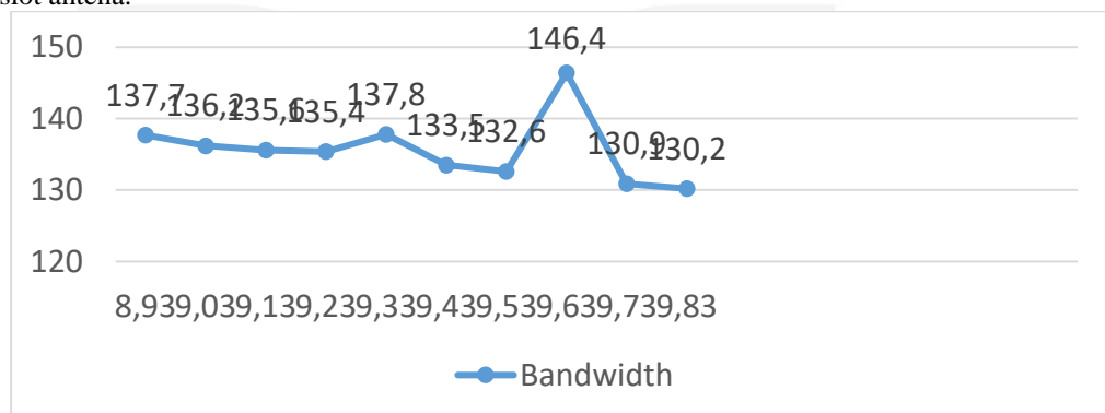
Gambar 6 Grafik Ls Nilai Bandwidth Antena Dengan Slot
