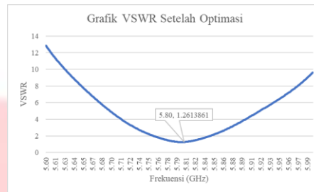
Gambar 3. 3 Grafik yang menunjukkan nilai VSWR dari simulasi hasil optimasi.
