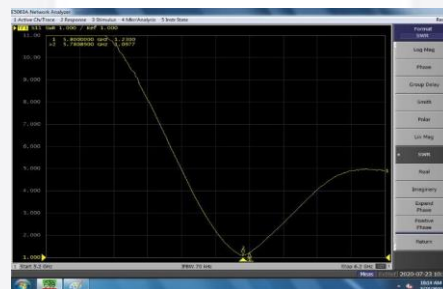
Gambar 4. 3 Pengukuran VSWR berdasarkan frekuensi.
