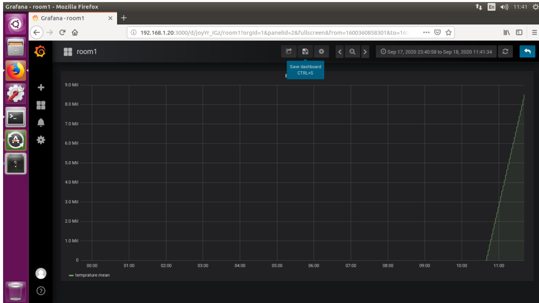
Gambar 3.8 Sistem Monitoring IoT menampilkan data Suhu
