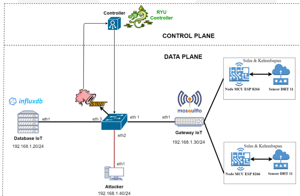
Gambar 3.1 Desain Sistem
