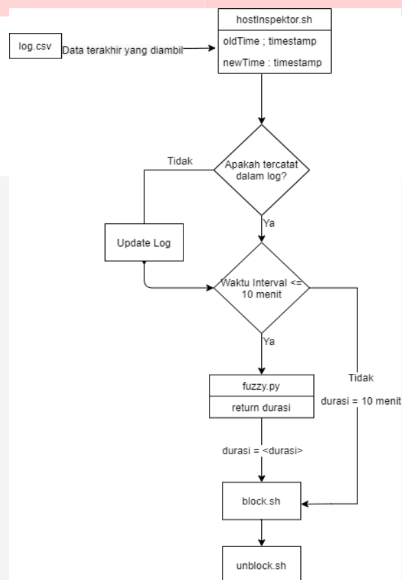
Gambar 3.3 Alur Cara Kerja Sistem
