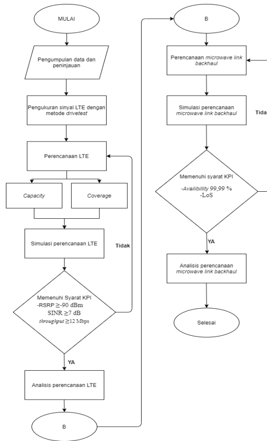
Gambar 3 Diagram alir perencanaan
